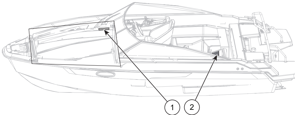
Figure 8.2 Yamarin 63 DC - Emplacement des panneaux de fusibles
