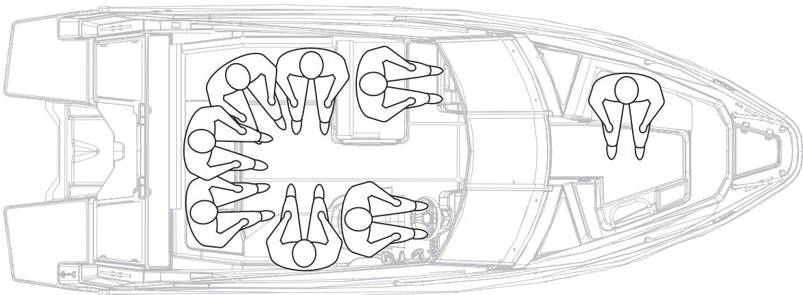
Figure 4.2 Yamarin 63 BR - Sièges pour un maximum de huit (8) passagers
