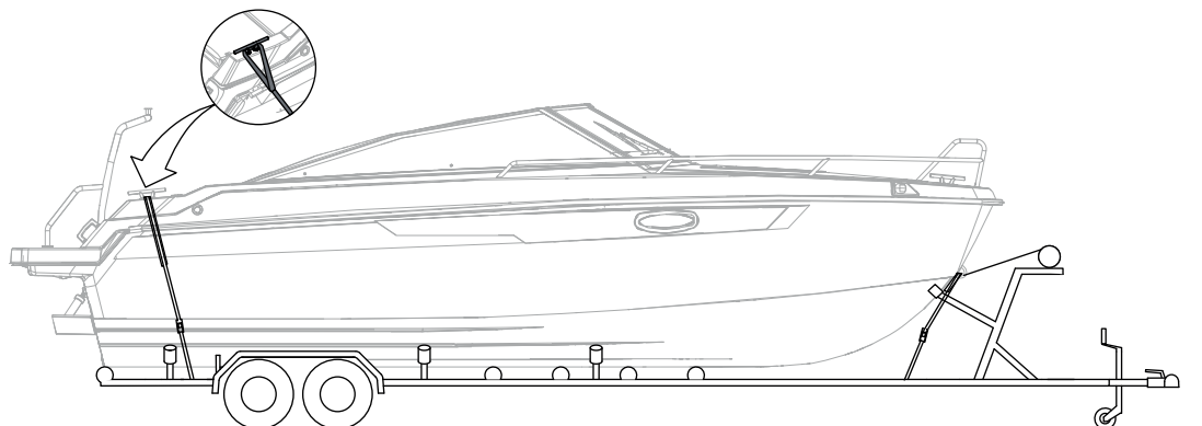
Figure 12.1 Yamarin 63 DC - Transport sur remorque
