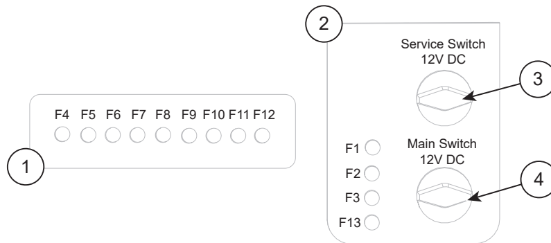
Figure 8.1 Yamarin 63 DC/BR - Interrupteurs principaux et panneau de fusibles
