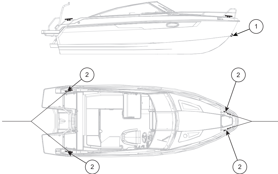
Figure 5.7 Yamarin 63 DC - Points d'amarrage et de remorquage
