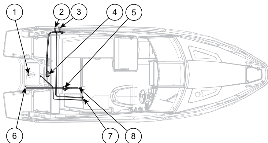
Figure 9.1 Yamarin 63 DC - Pompes et vidange de cale
