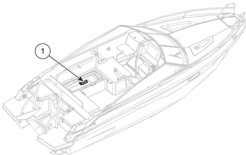
Figure 2.2 Yamarin 63 DC - Emplacement de l'extincteur
