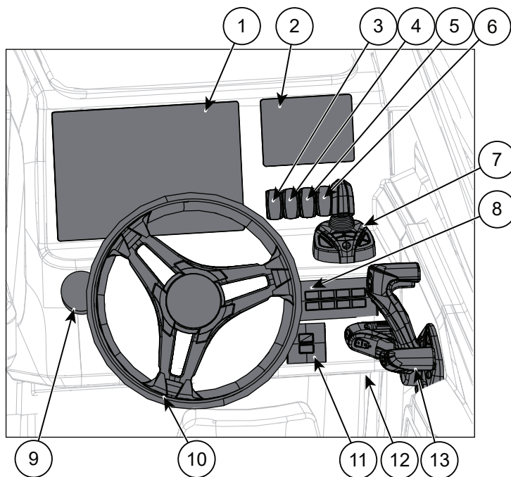
Figure 5.1 Yamarin 63 DC/BR - Commandes du poste de barre
