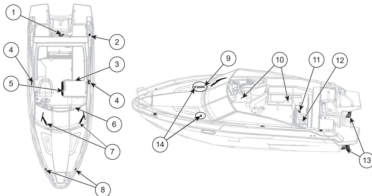
Figure 8.4 Yamarin 63 DC - Équipement électrique
